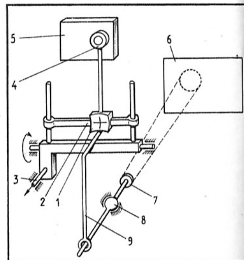
РИС. 2. Схема устройства для наведения фотоприемника на изображение сюжетно-важного объекта при компоновке кадра: 1 — передвигаемый поводок; 2 — координатные направляющие; 3 — спусковая кнопка; 4 — ограничительный кружок; 5 — поле зрения видоискателя; 6 — кадровое окно фотоаппарата; 7 — фотоприемник системы «прямого измерения»; 8 — шаровая опора; 9 — рычаг (для поворота фотоприемника 7 при перемещениях поводка 1)
